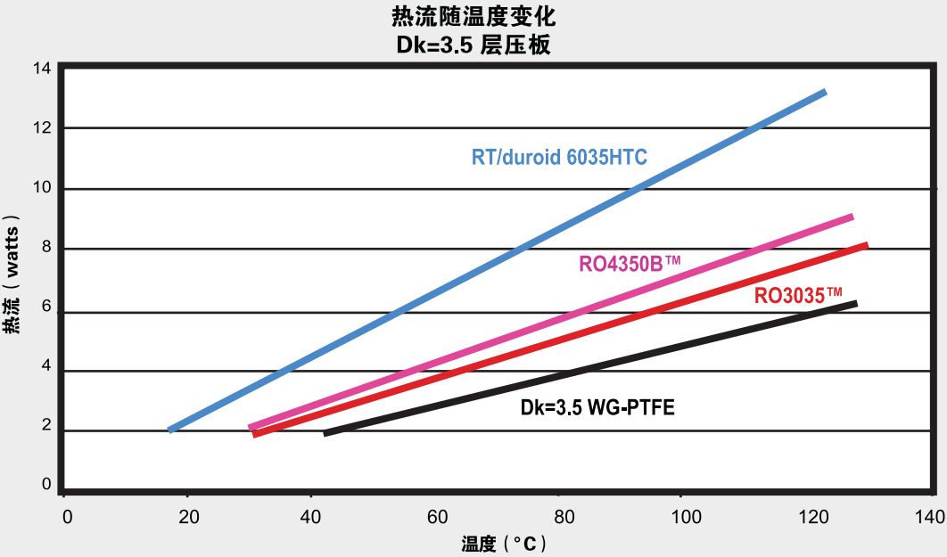
图1. 测试四个Dk为3.5的不同层压板材料，RT/duroid 6035HTC电阻散热效率最高，温度上升最慢
