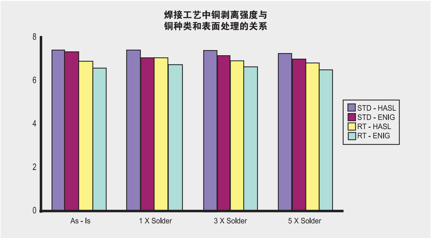
图2. 描述了耐受288℃(550°F)高温焊接60秒的0.125"宽度铜箔线路的剥离强度，罗杰斯RT/duroid 6035HTC的铜箔在多次高温焊接条件下表现出卓越的热稳定性，确保了高功率、高工作温度下设备的长期稳定性。
